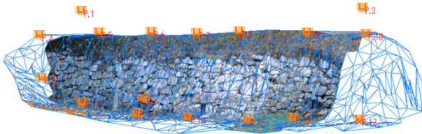
図-8 イメージ・ベスト・モデル手法による正射投影写真
