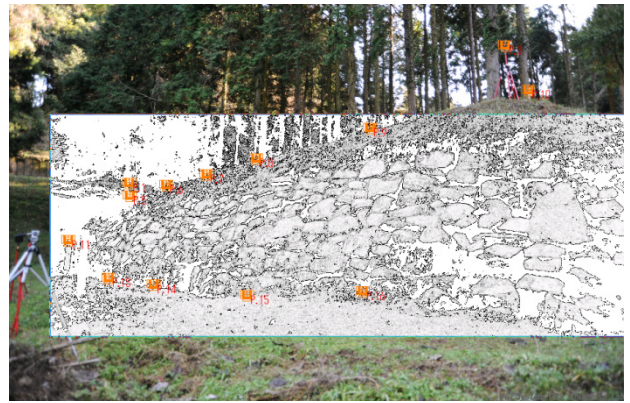
図-9 エッジ処理を施した写真画像
